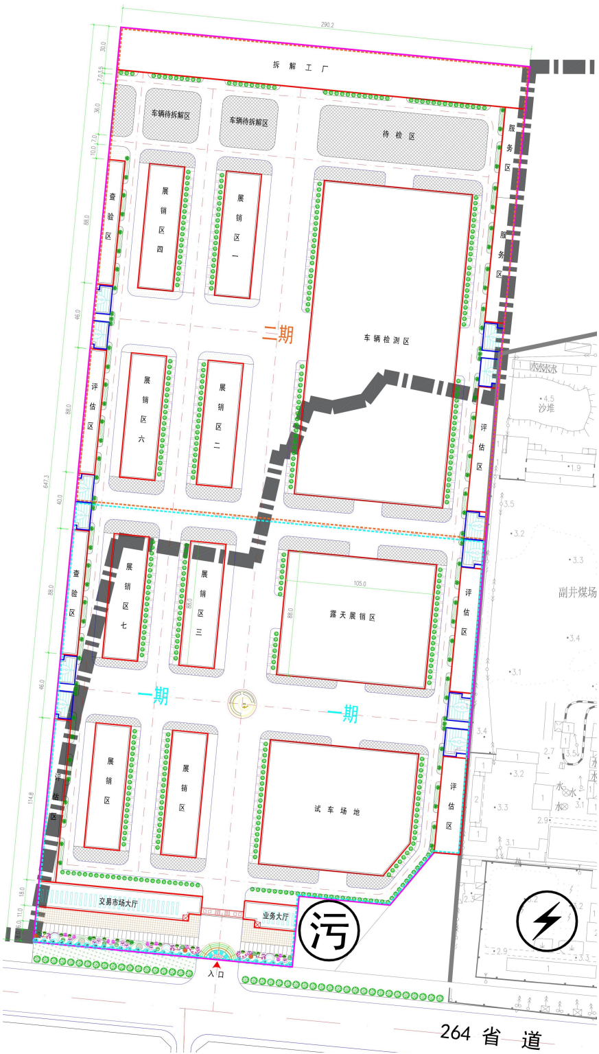
附图 7: 龙口市新材料科技产业园绿色智能二手车交易中心平面图
